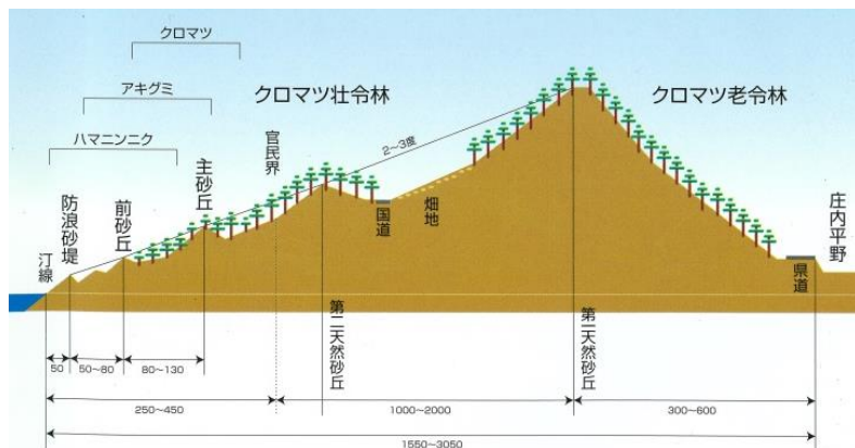
庄内砂丘の一般的な横断面図
