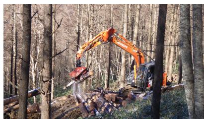
高性能林業機械を使用した 低コスト施業
