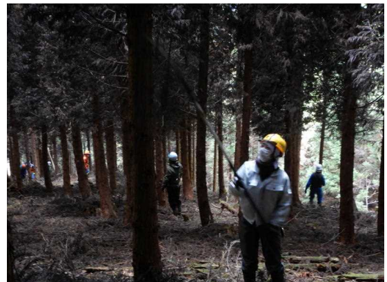
高枝用のこぎりによる枝打ちの様子
