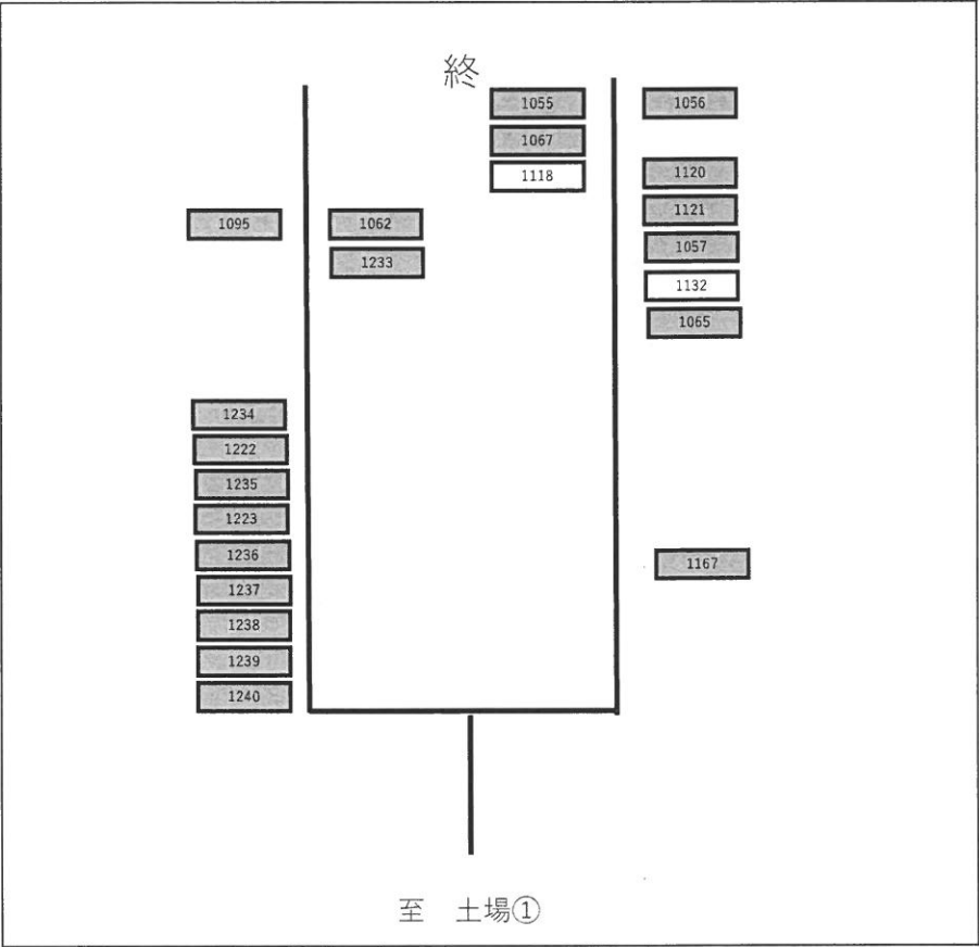
巻立位置図
