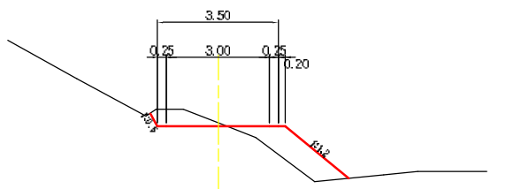
標準断面図 S=1:100
