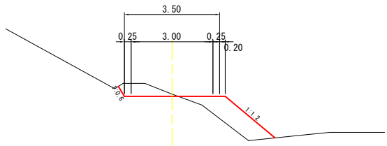
標準断面図 S=1:100
