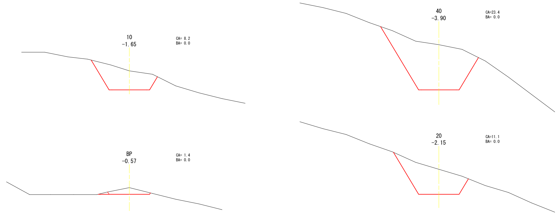
重機進入路横断面図 S=1:100
