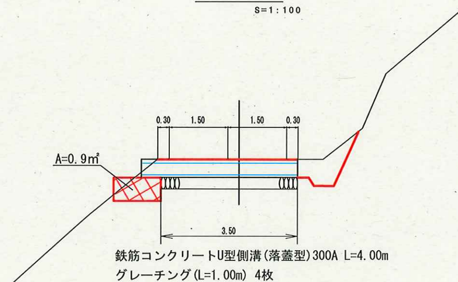
4.8km地点 S=1:100
