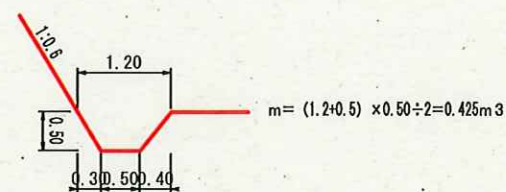
大型側溝標準図 S=1:100
