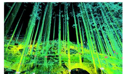
地上型3Dレーザを活用した調査（イメージ）
