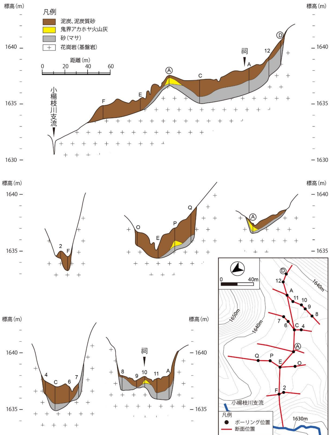
図8 花之江河のボーリング調査から推定される湿原堆積物の推定縦断面図と推定横断面図 各地点におけるボーリングコア試料の柱状図は図9を参照されたい。
