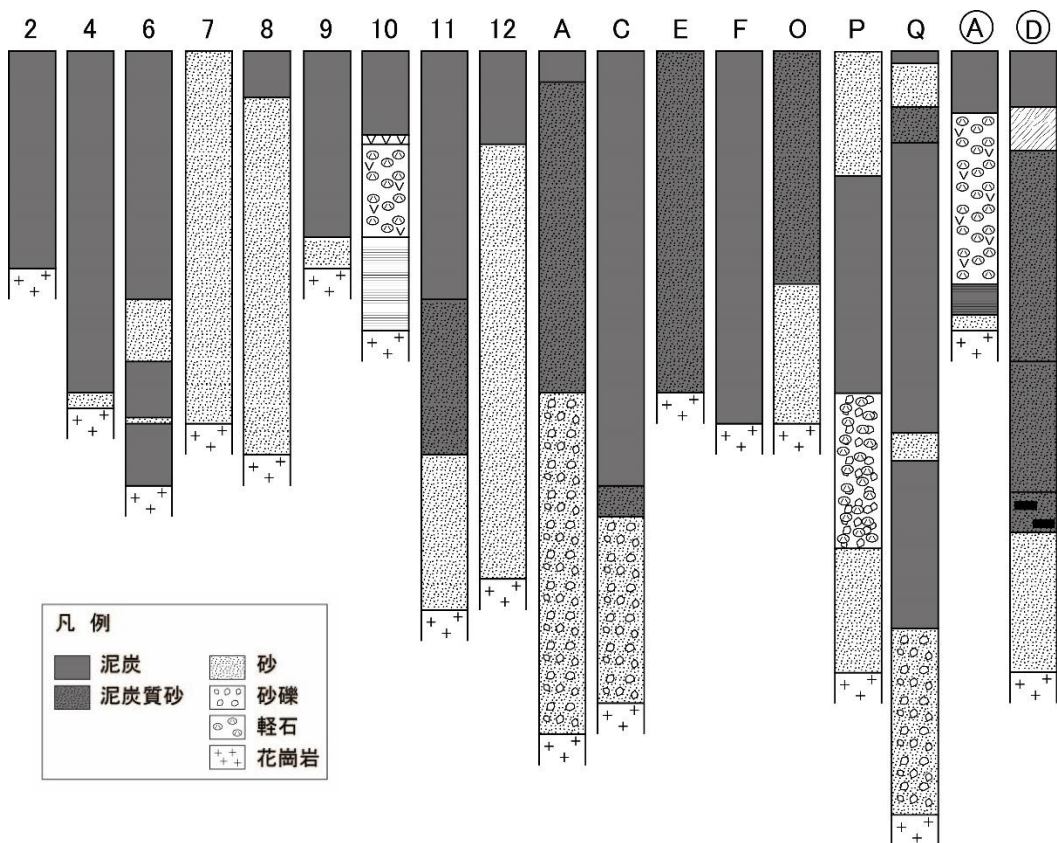
図9 花之江河におけるボーリングコア試料の柱状図
