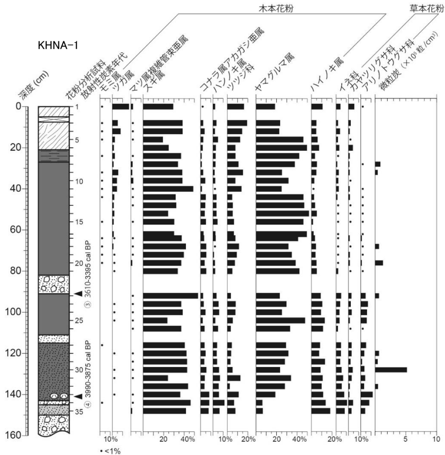
図 12 小花之江河 (KHNA-1) における主要花粉分析組成図と微粒炭濃度
