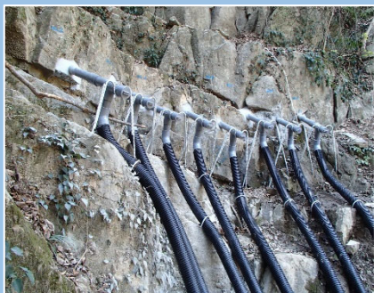
ボーリング暗きょ工
