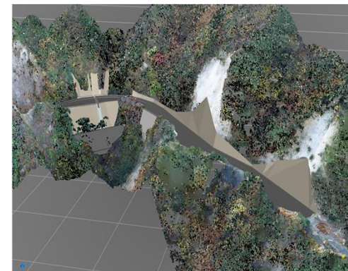
林道改良工事個所の3次元モデルと地形データ (敦賀市：黒河林道アシ谷支線)
