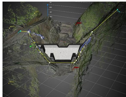
溪間工事の3次元モデルと地形データ (若狭町：河内溪間工事) こうち
