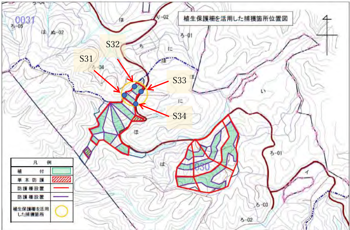
図 10 植生保護柵への扉の設置位置
