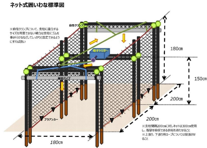
図 3-1 ネット式囲いわな標準図
