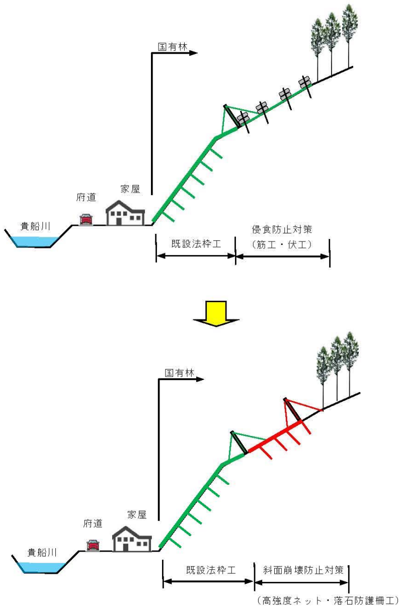
山腹工Cタイプ模式図
