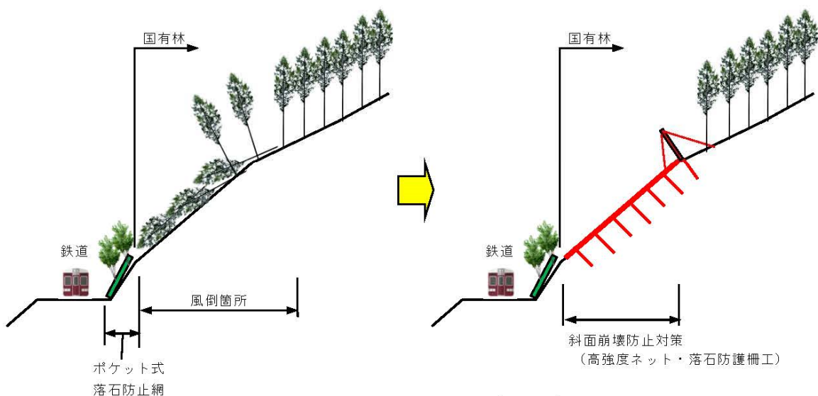
山腹工 A タイプ模式図 (計-14)
