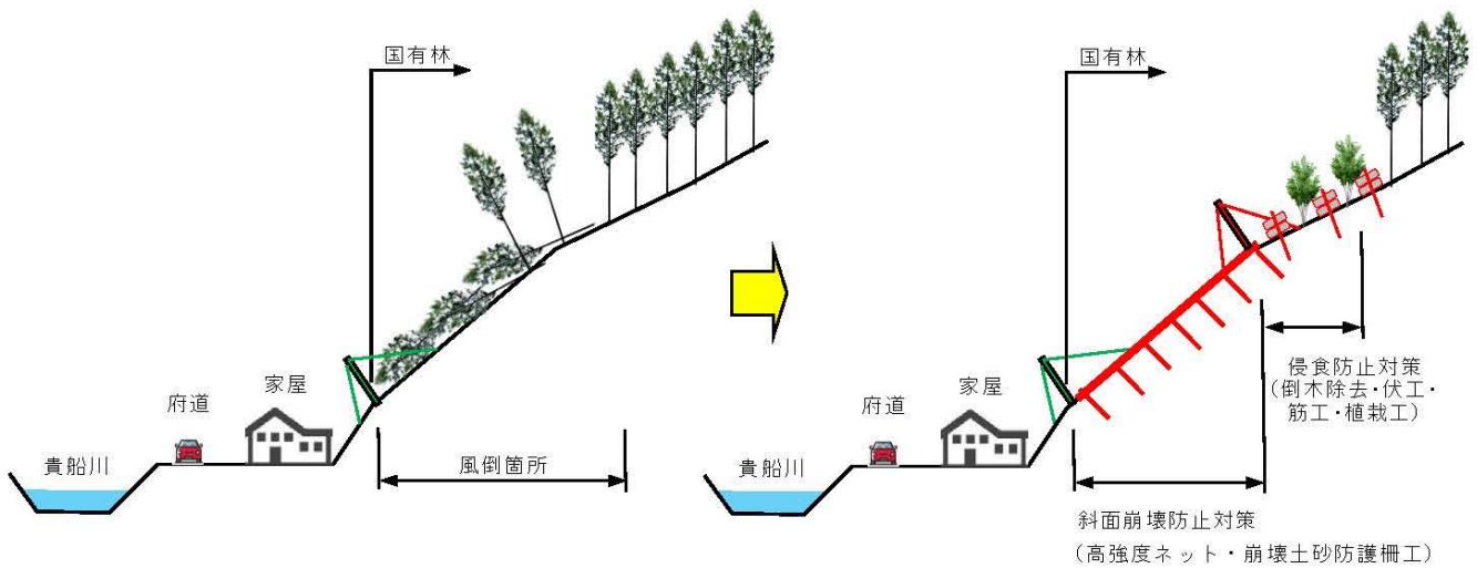
山腹工 A タイプ模式図 (計-10)
