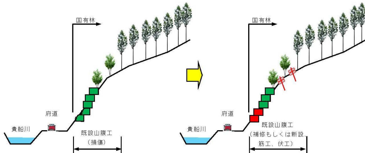
山腹工Dタイプ模式図
