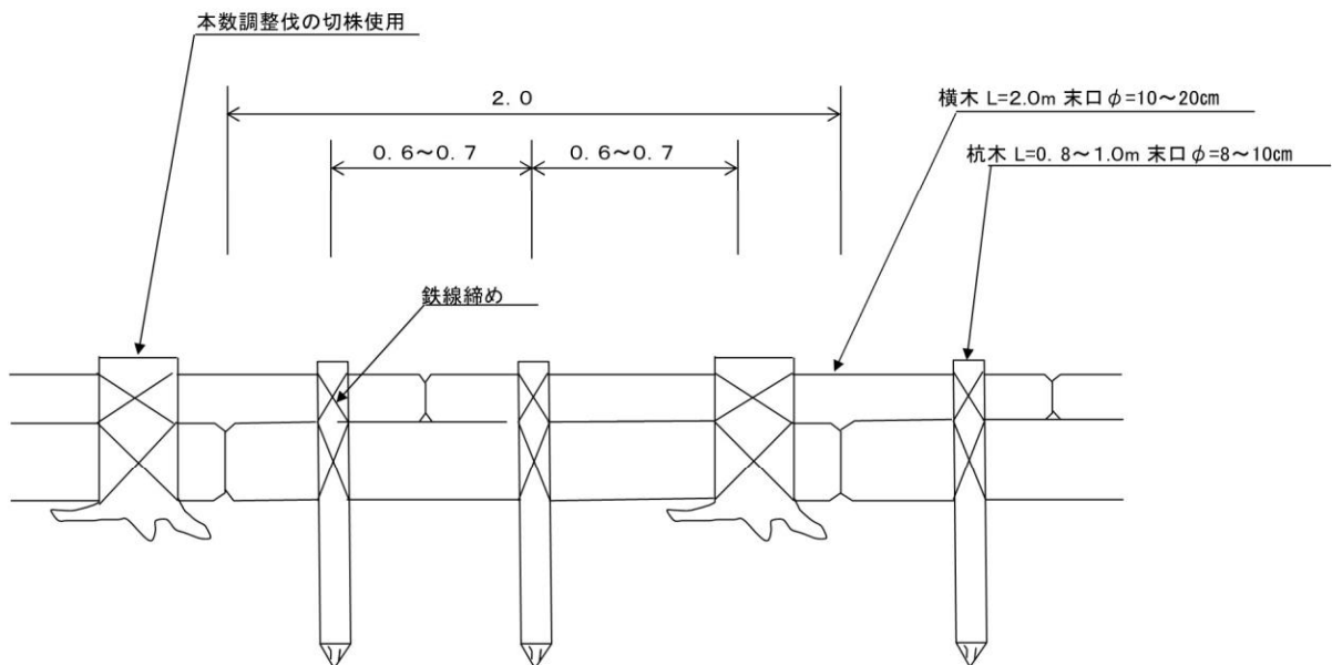
断面図
