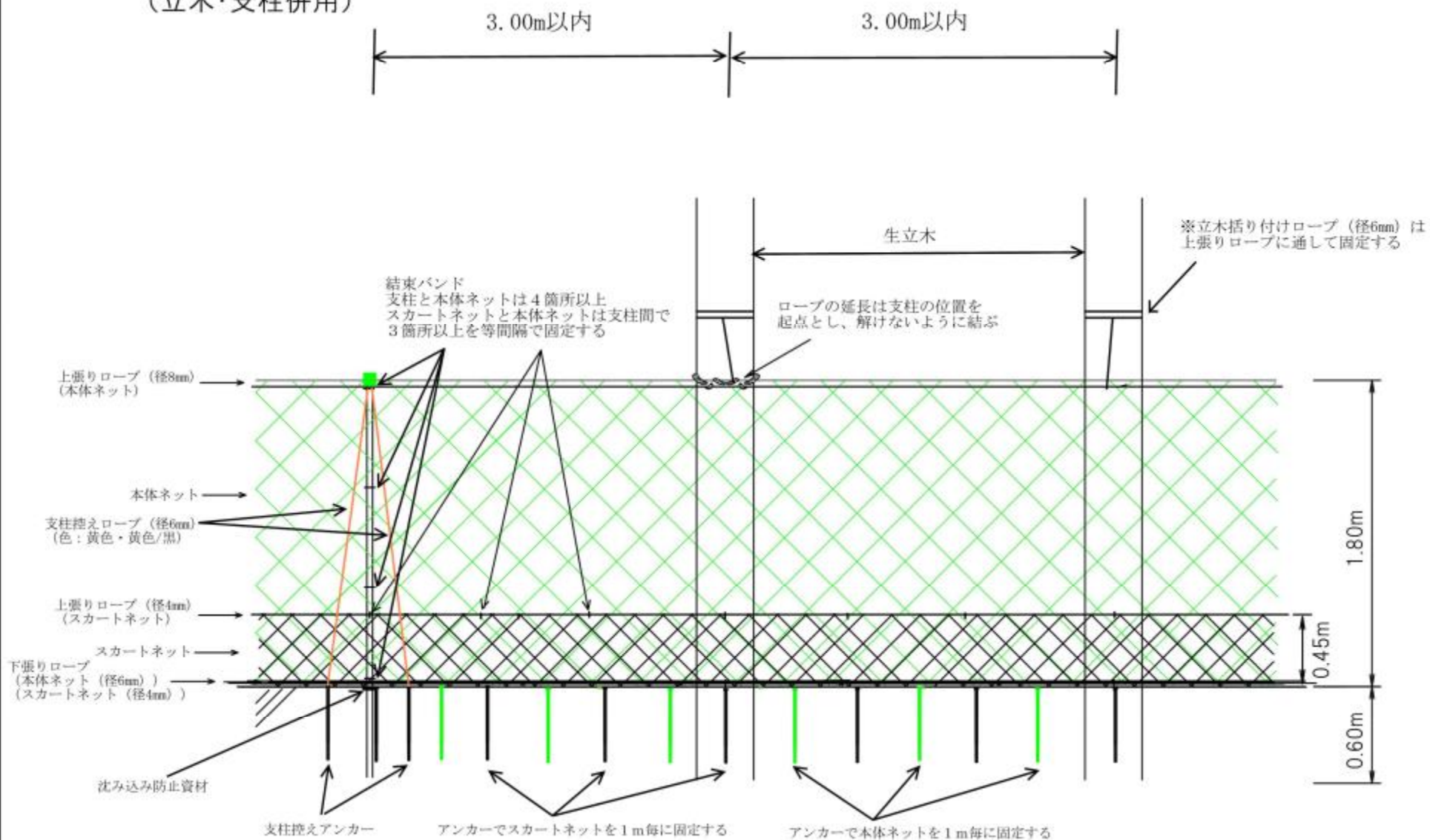
防護柵標準図 1 (立木・支柱併用)
