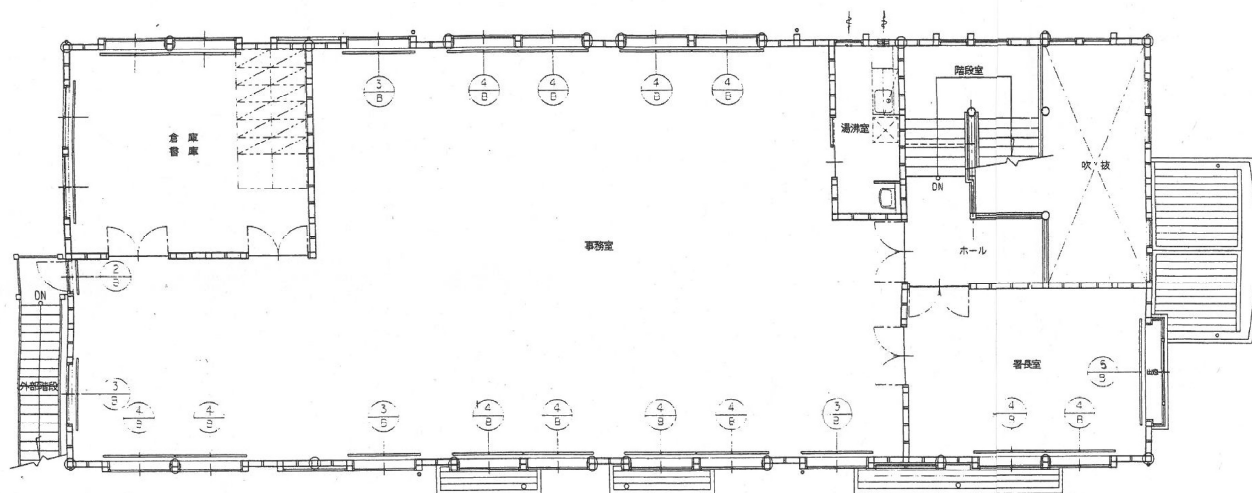
2階 平面図
