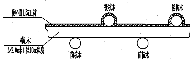
平面図
