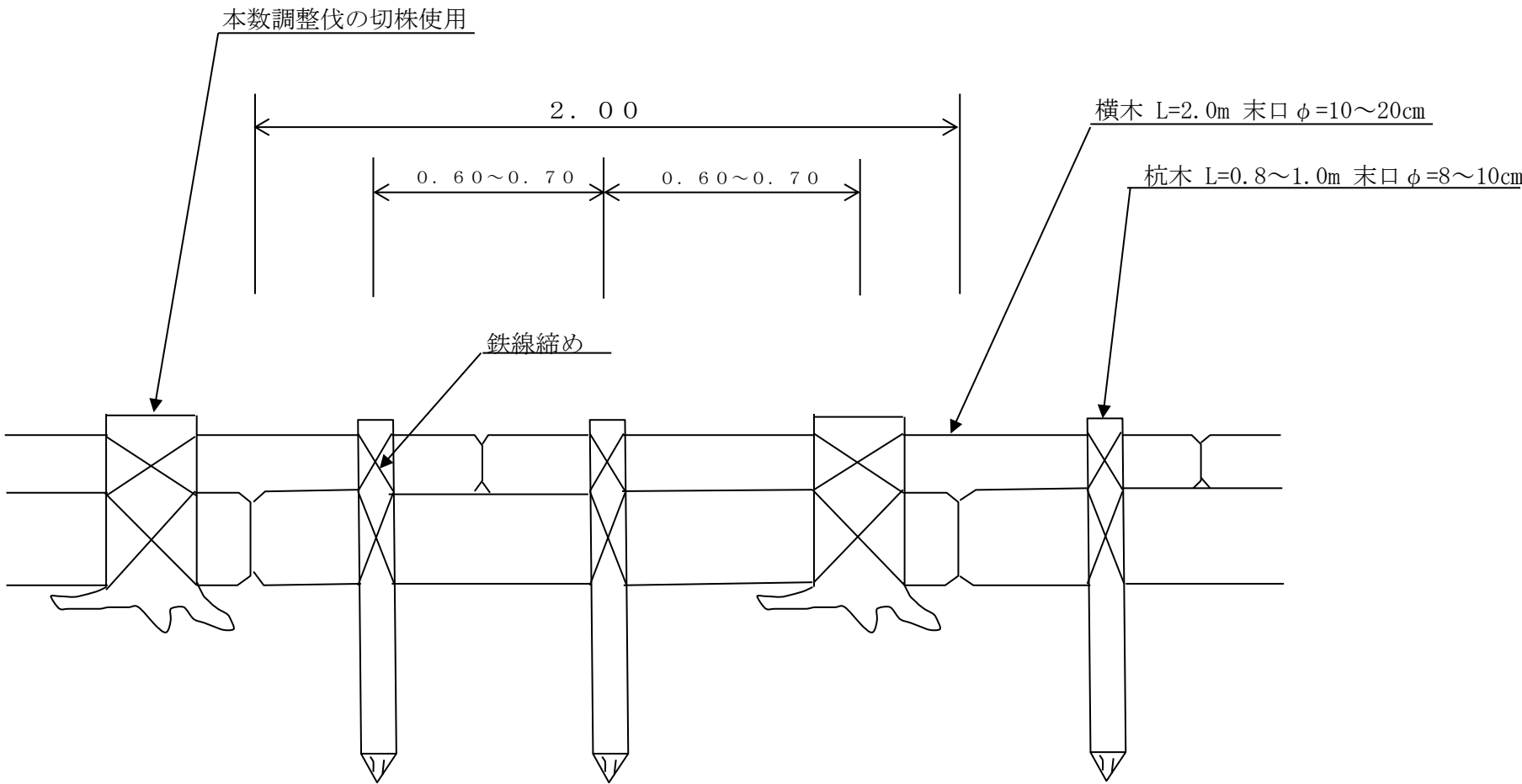
正面図
