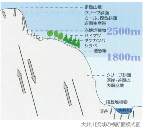
大井川流域の横断面模式図
