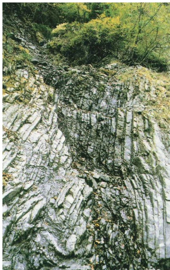
褶曲・節理の発達した地質
