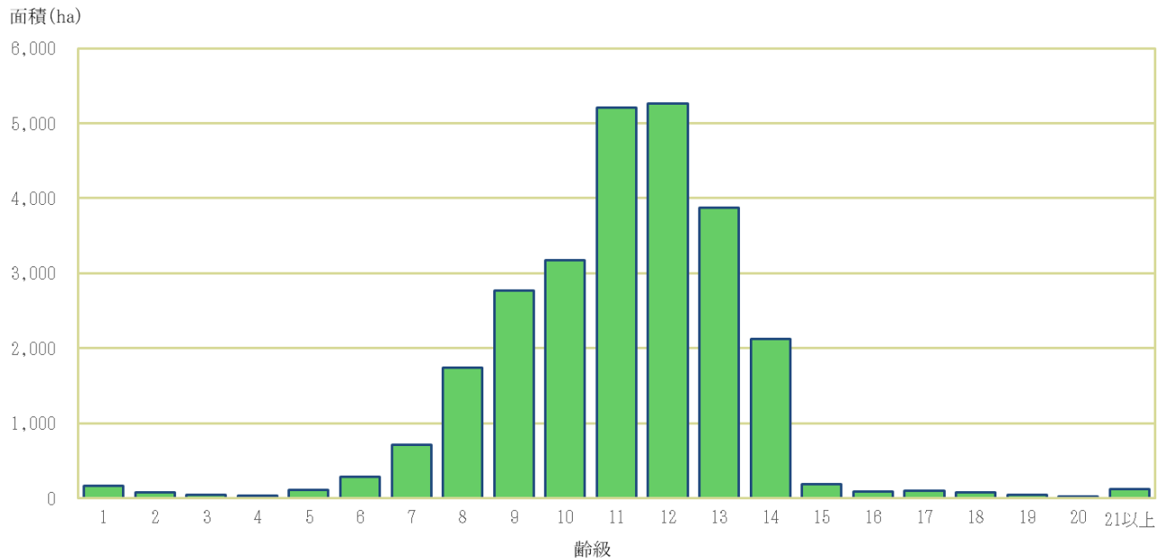
図－4 人工林の齢級構成
