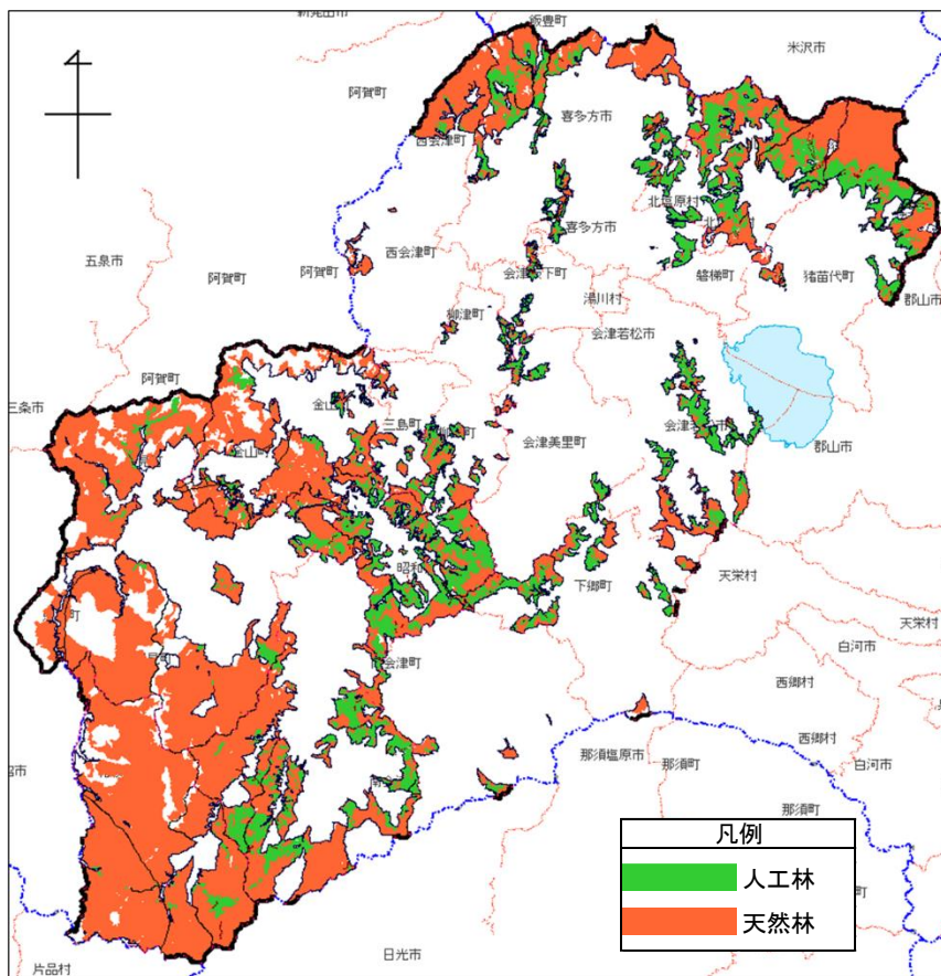
図－2 人工林、天然林の分布状況
