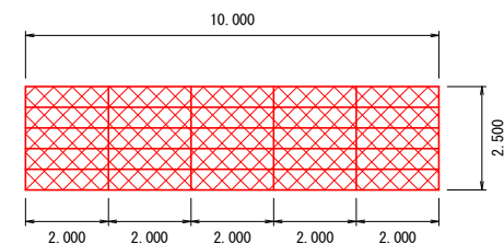
ふとん籠工 展開図
