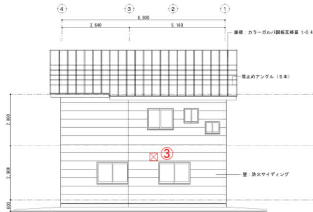
北立面図 S=1/100
