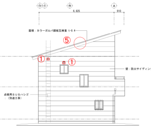
西立面図 S=1/100
