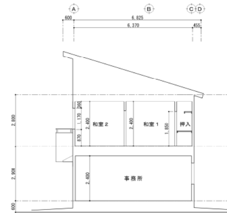
B-B'断面図 S=1/100
