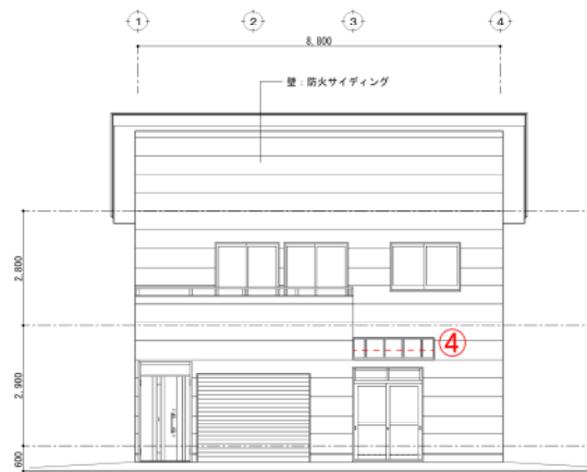
南立面図 S=1/100
