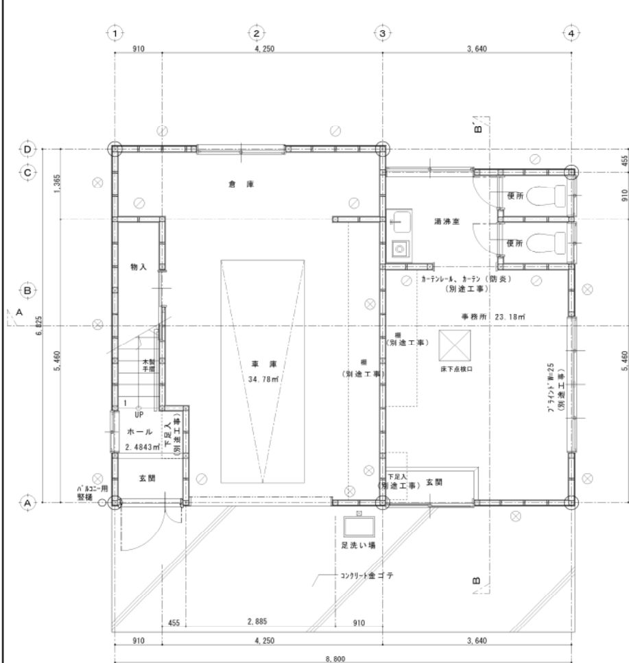
1 階 平 面 図 1 : 5 0
