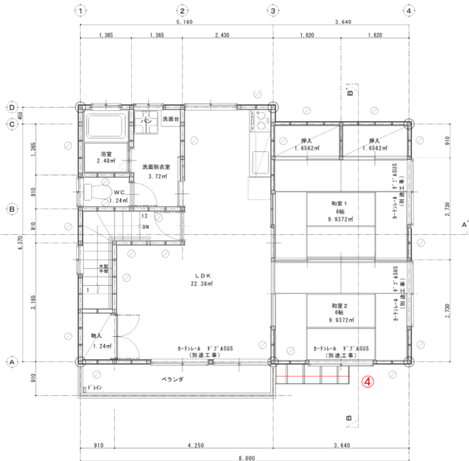
2 階 平 面 図 1 : 5 0
