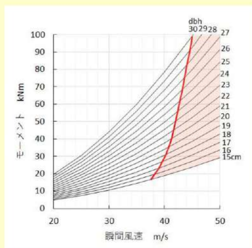
dbhと根張り風速
