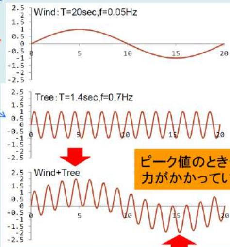
図14 樹木の揺れの模式図
