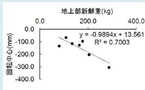
回転中心の深さと地上部重量
