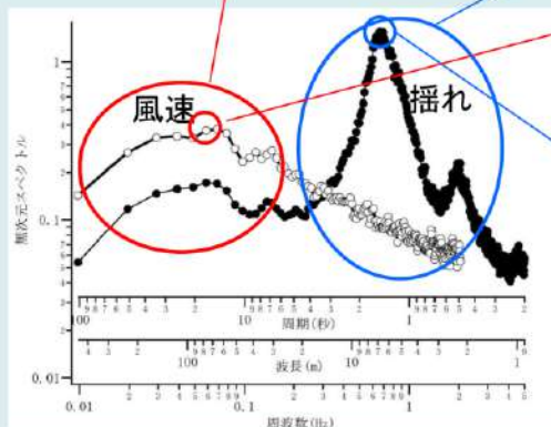
図13 樹木の揺れと風速(5年生スギ)
