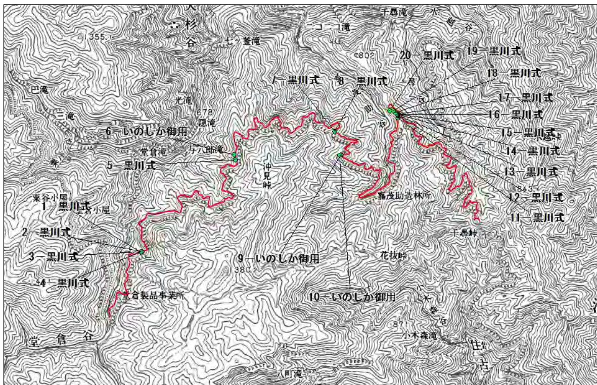
図 2.2.9 くくりわな設置位置
