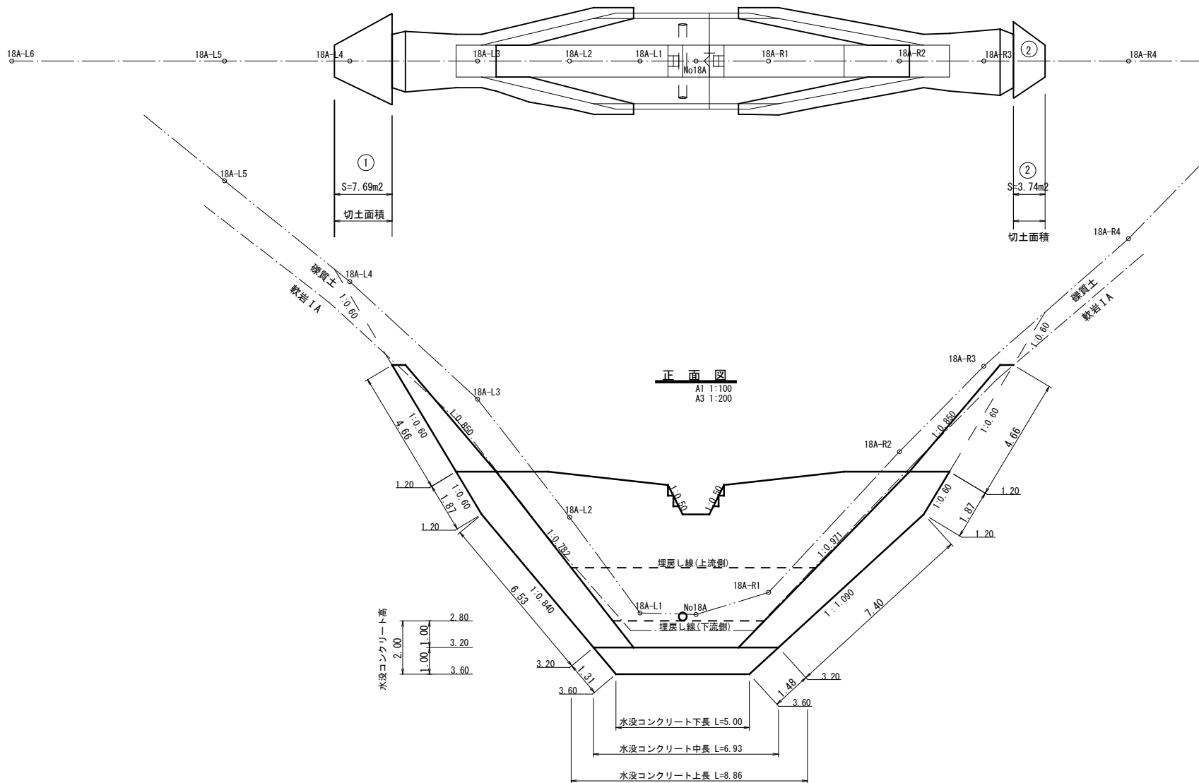
緑化範囲 平面図 A1 1:100 A3 1:200
