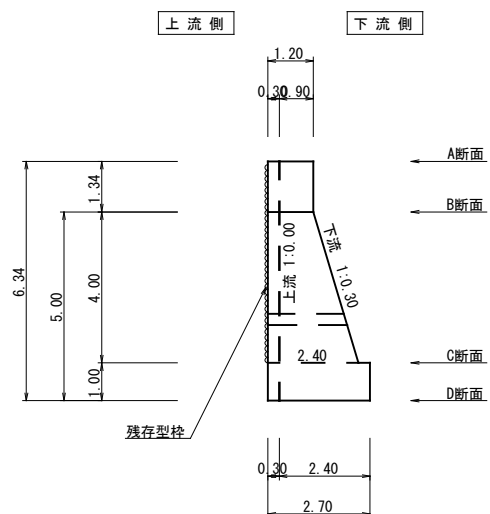
伸縮継目1平面図
