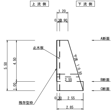
伸縮継目1 断面図 A1 1:100 A3 1:200
