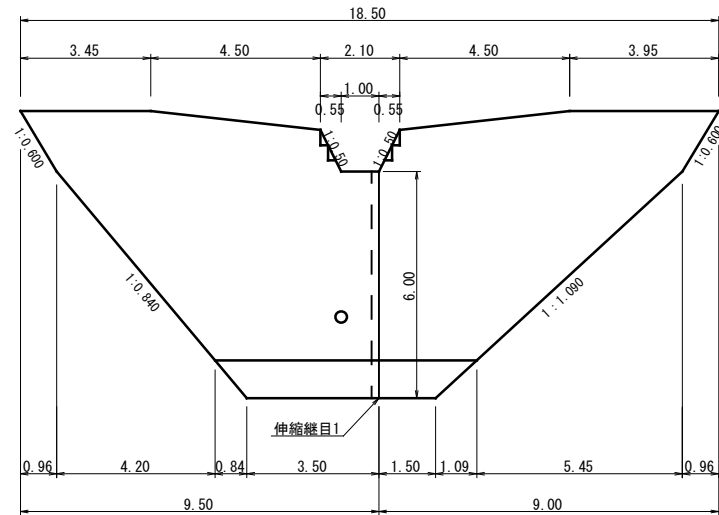
正面図 A1 1:100 A3 1:200
