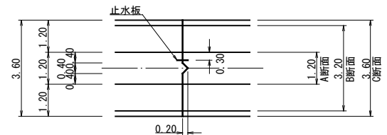
伸縮継目1平面図 A1 1:100 A3 1:200
