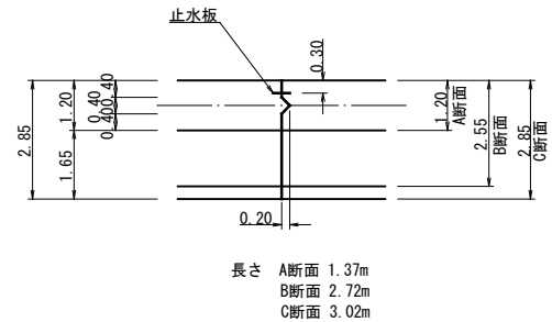
伸縮継目1平面図 A1 1:100 A3 1:200
