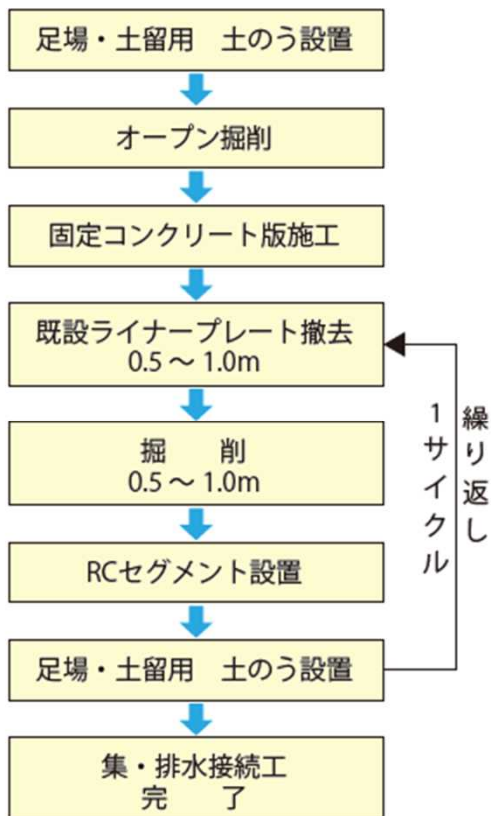
（セグメントブロックの設置）
