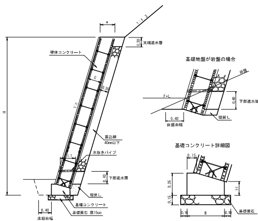
寸法表
