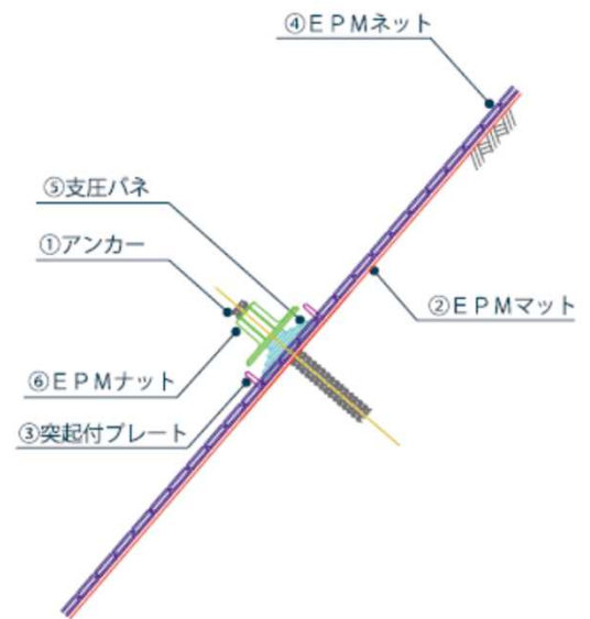
A部断面図
