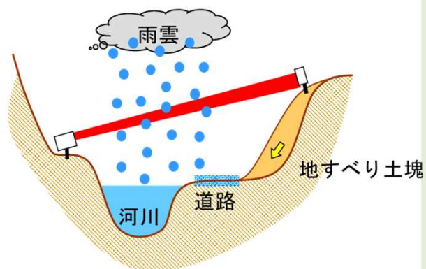
拡散レーザー変位計の場合
