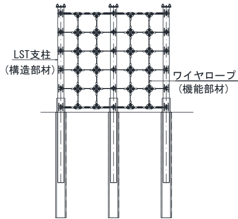
アーバンガード構造図
