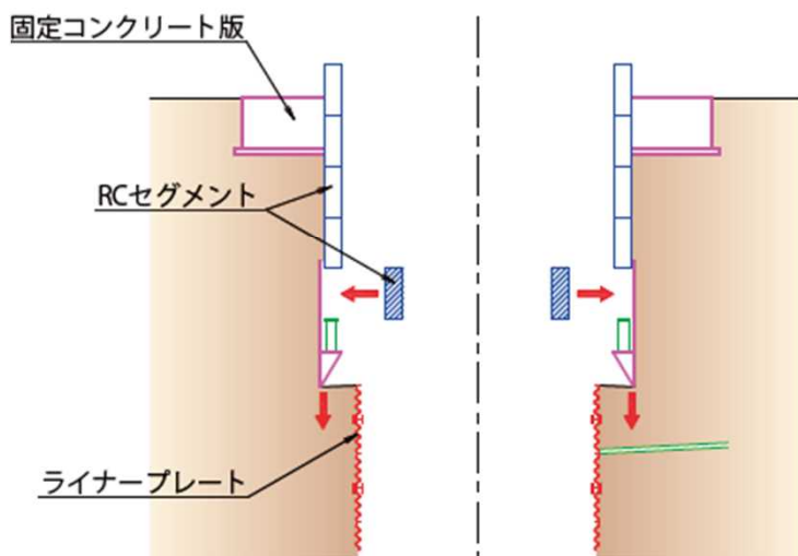
（ジャッキによる刃口押上げ）
