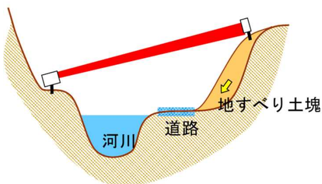
拡散レーザー変位計の場合
