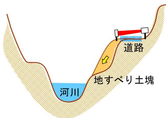
拡散レーザー変位計の場合
